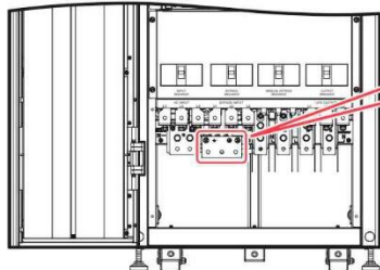
Рисунок 2-10: клеммы заземления
