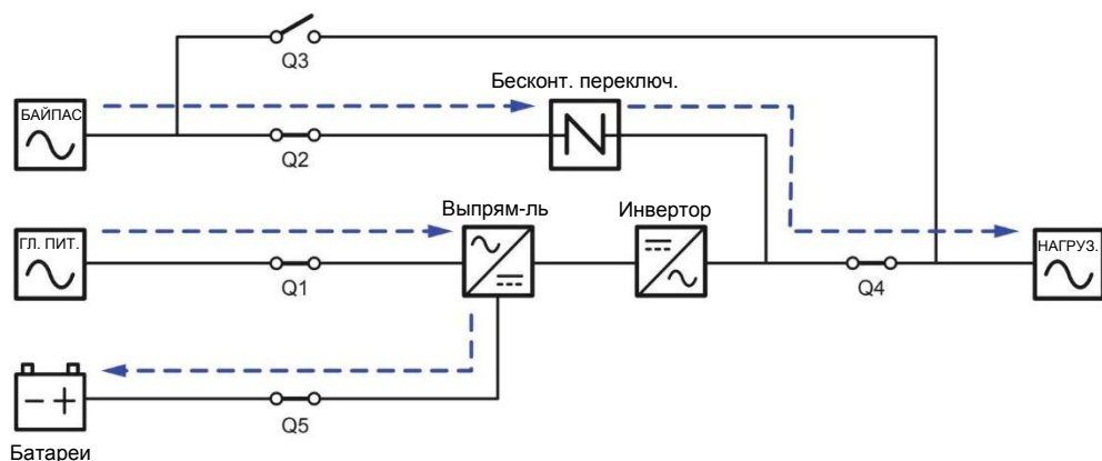
Рисунок 3-17: схема байпасного режима, подключение одного ИБП к двум линиям
